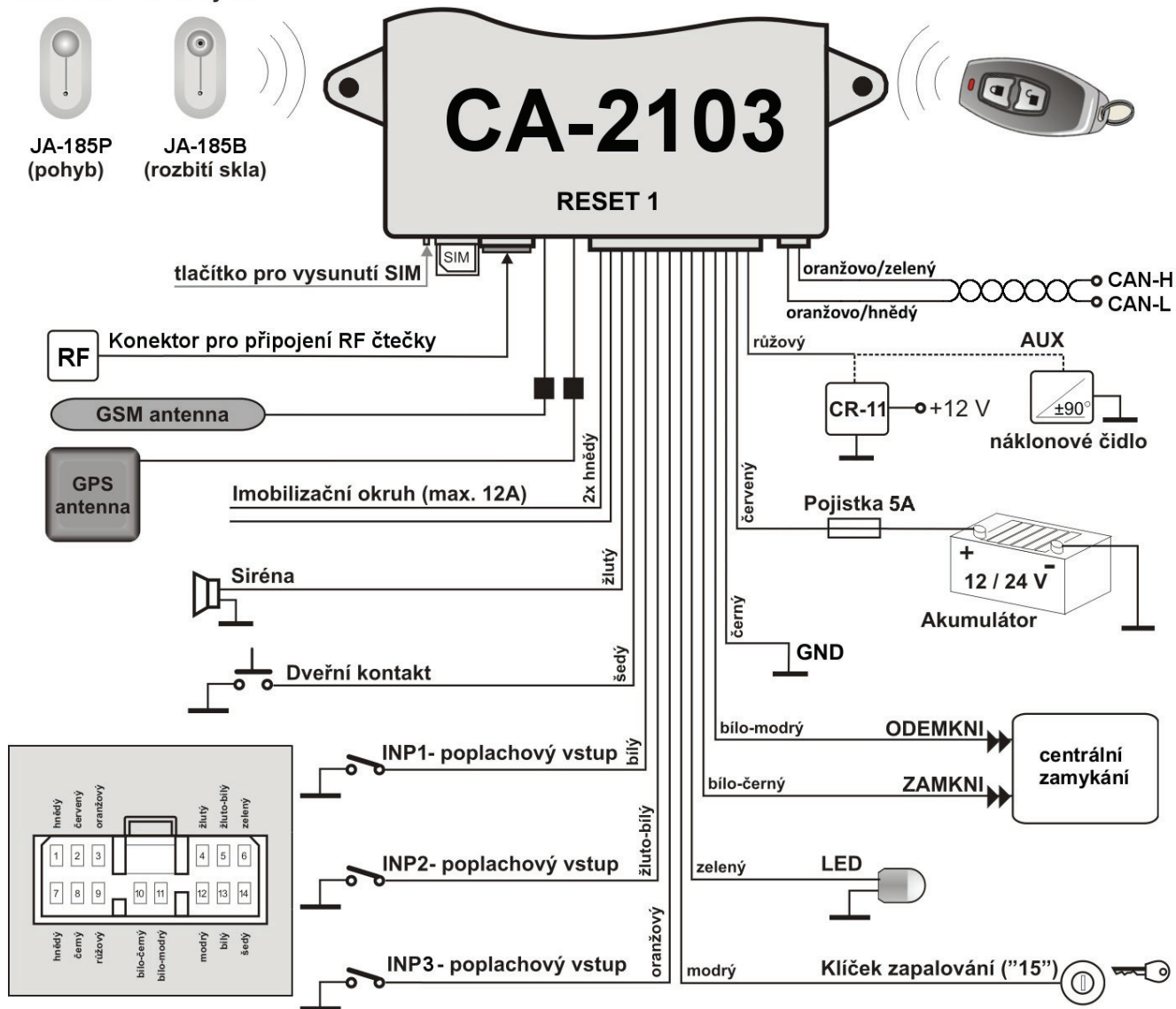
Obr. 1: Zapojení alarmu v profilu RESET 1. V tomto zapojení je autoalarm schopen ovládat centrální zamykání vozu.
