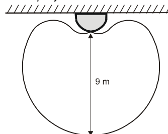
detekční pokrytí detektoru – pohled shora či z boku
